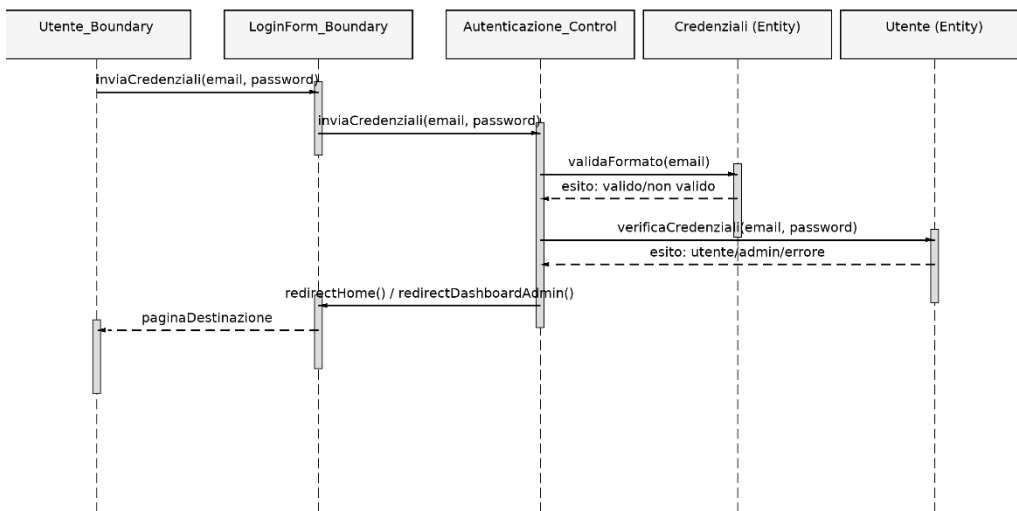
Sequence Diagram - UC1 Autenticazione
