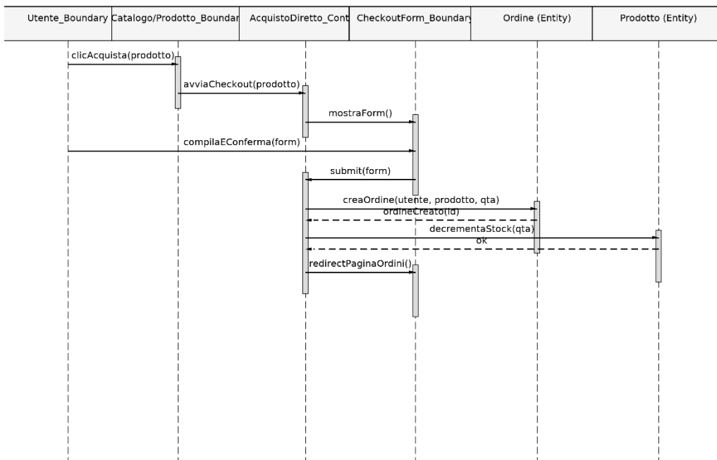
Sequence Diagram - UC3 AcquistoDiretto
